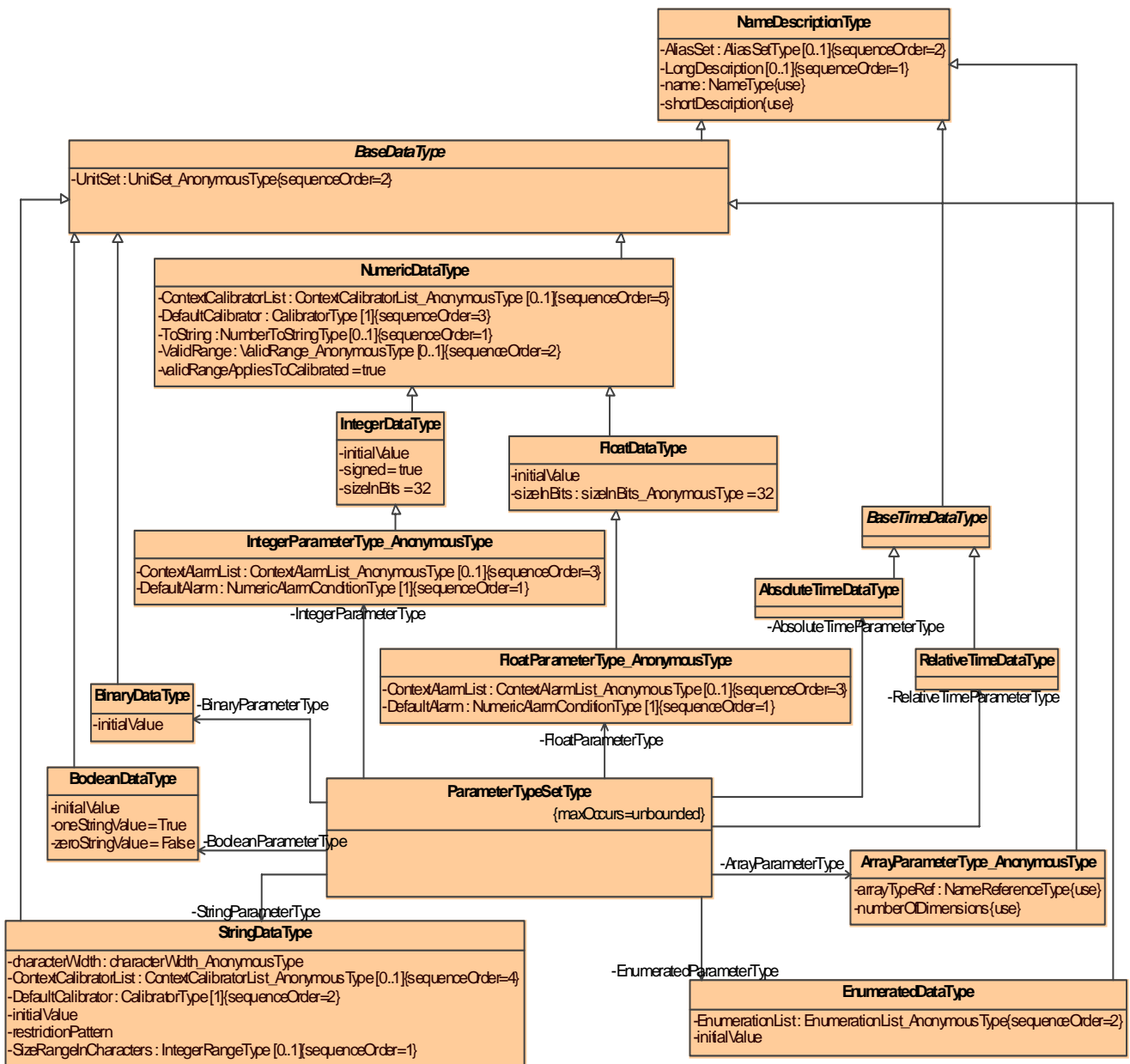
Figure 7.3 - ParameterTypeSet
