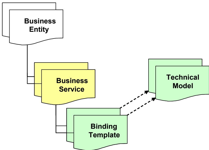
Figure 4: UDDI Overview
