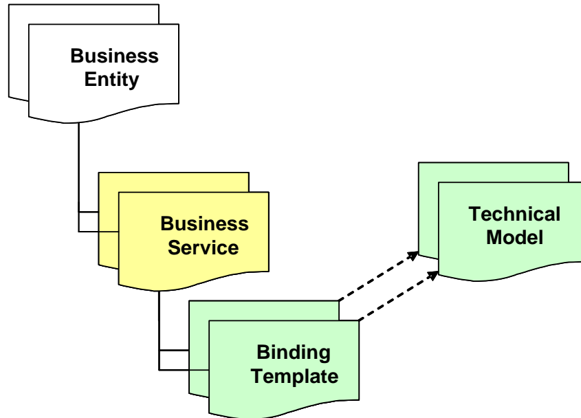
Figure 4: UDDI Overview
