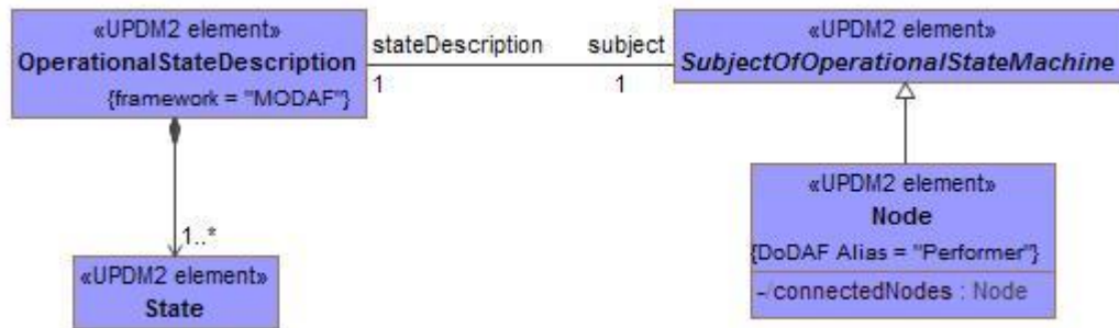
Figure A:14 - OV-6b - DMM
