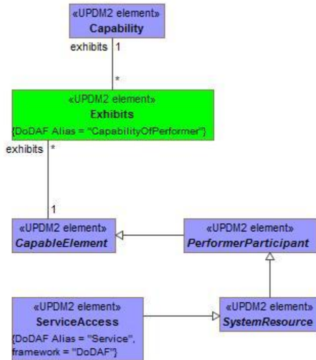
Figure A:24 - CV-7 - DMM
