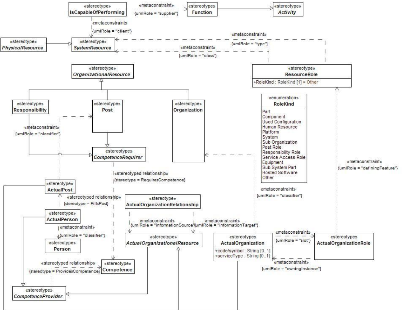
Figure B:12 - OV-4 Actual
