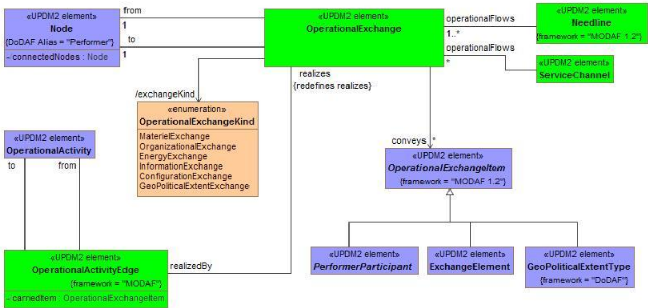
Figure A:9 - OV-3 - DMM
