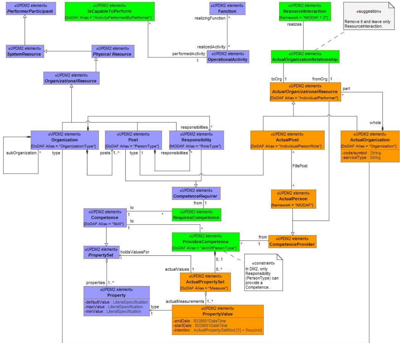
Figure A:10 - OV-4 Actual - DMM
