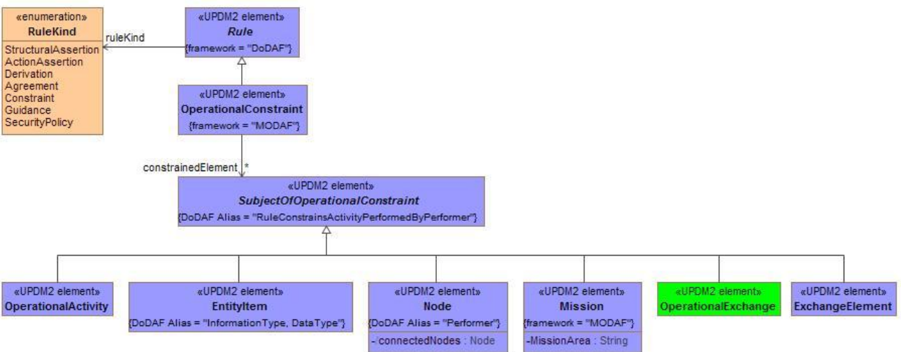
Figure A:13 - OV-6a - DMM
