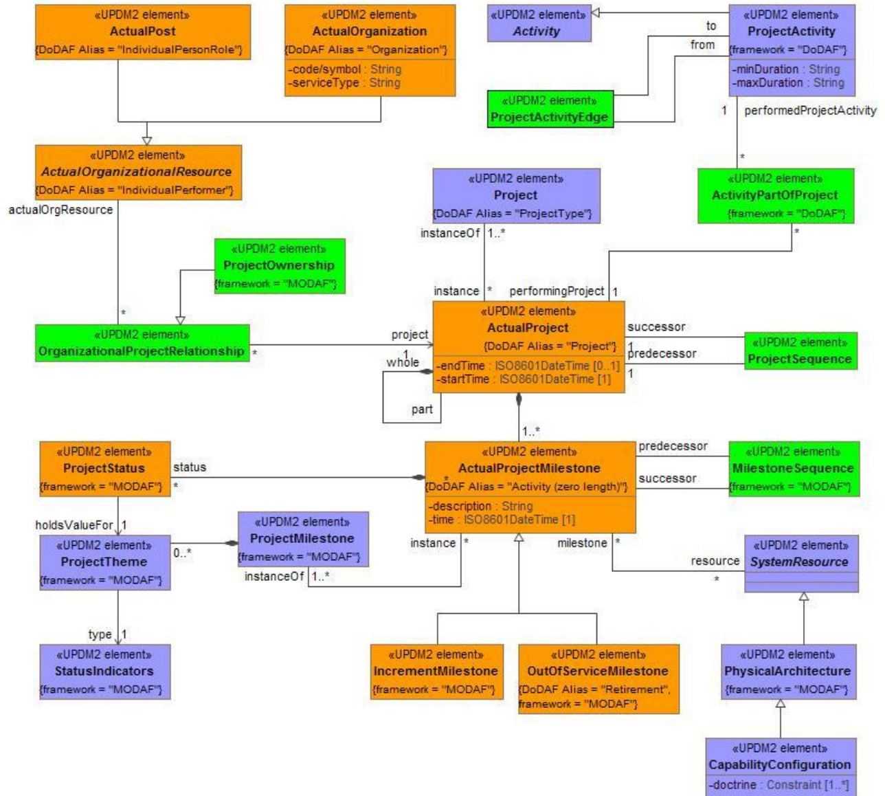
Figure A:2 - AcV-2/PV-2 - DMM
