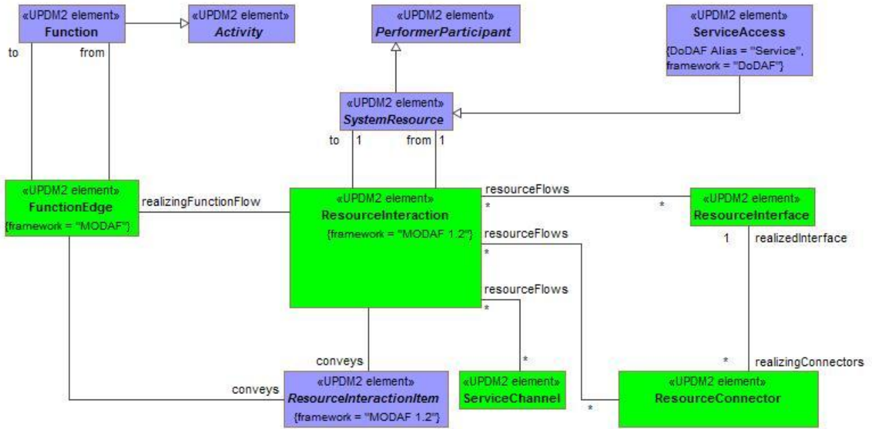
Figure A:41 - SV-6/SvcV-6 - DMM
