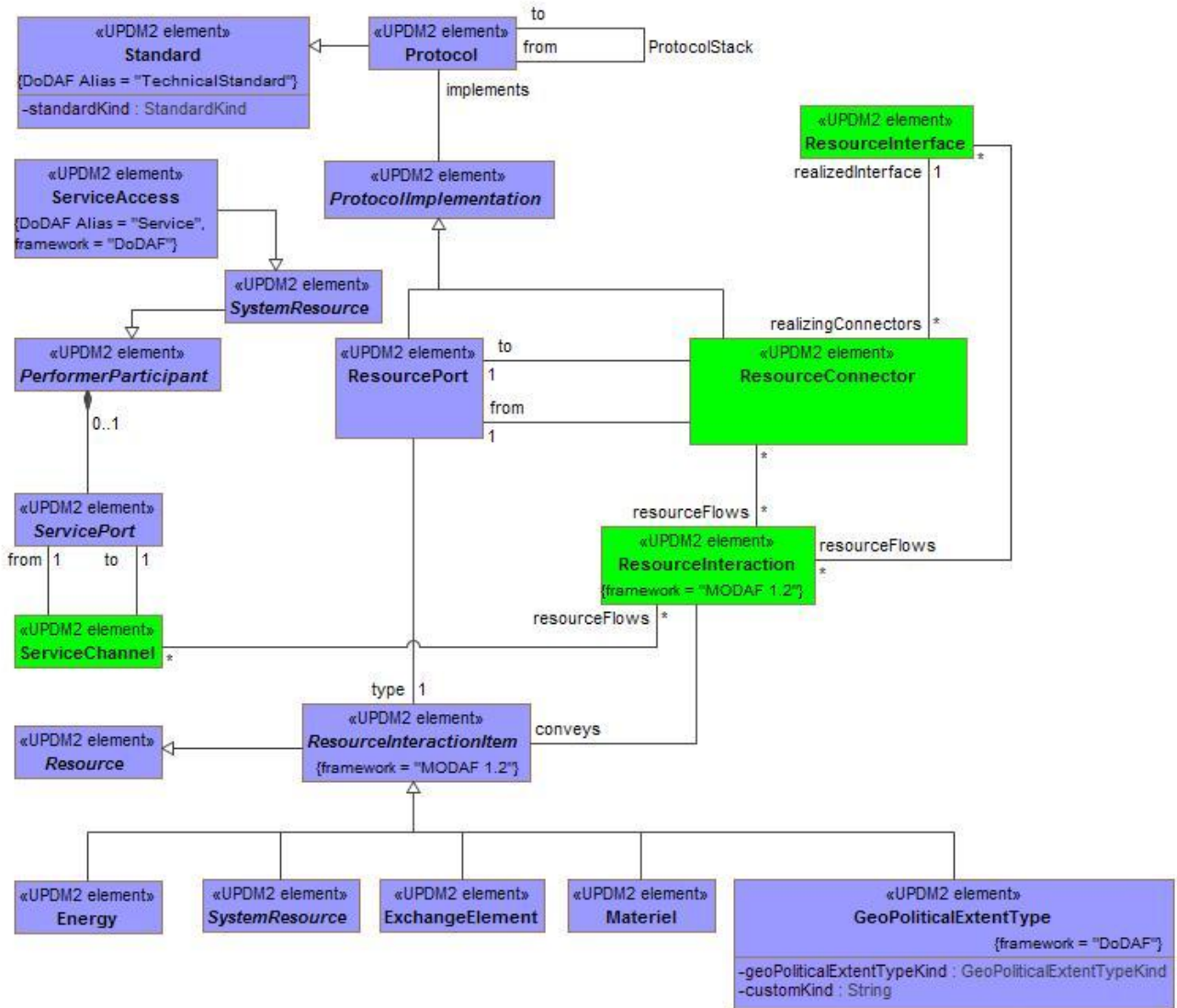
Figure A:37 - SV-2/SvcV-2 - DMM
