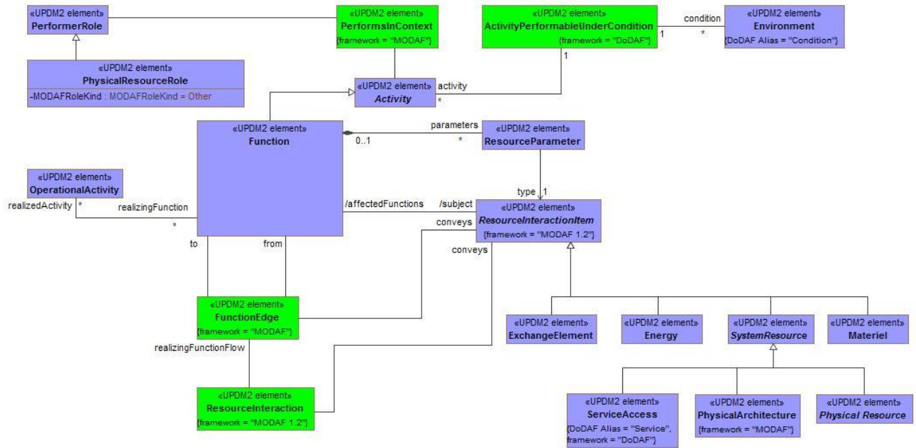
Figure A:38 - SV-4/SvcV-4 - DMM
