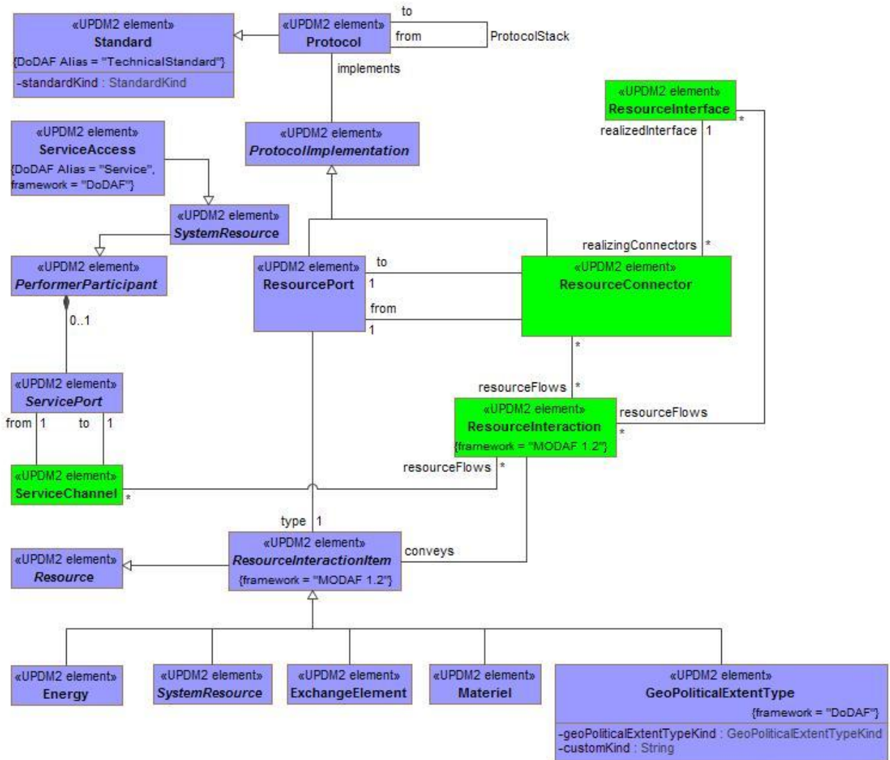
Figure A:36 - SV-2/SvcV-2 - DMM
