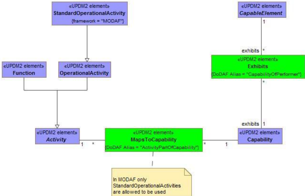
Figure A:29 - StV-6/CV-6 - DMM
