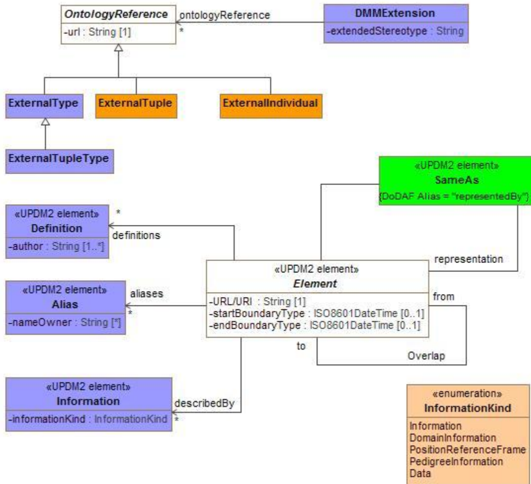
Figure A:5 - AV-2 - DMM
