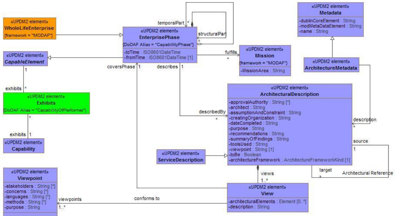
Figure A:4 - AV-1 - DMM
