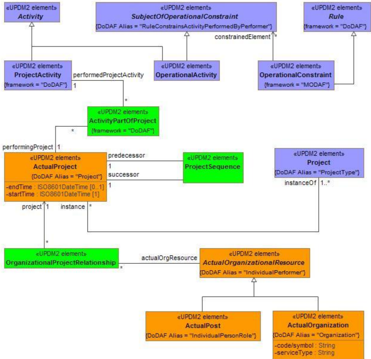
Figure A:56 - Project - DM2
