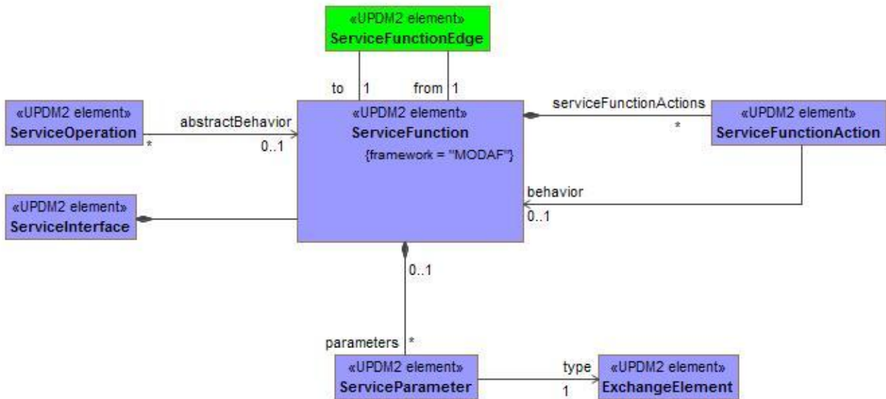
Figure A:22 - SOV-5 - DMM
