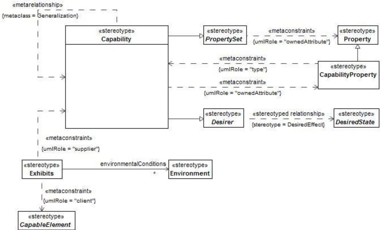
Figure B:27 - StV-2/CV-2
