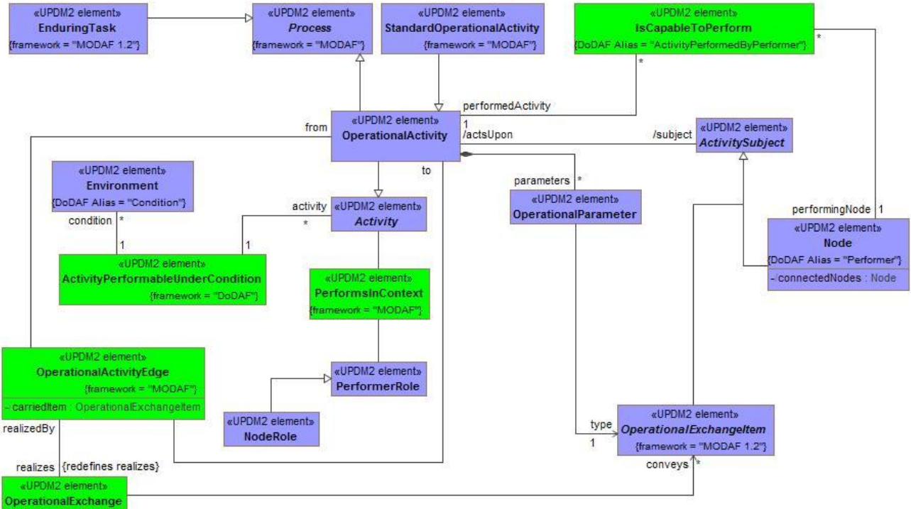
Figure A:11 - OV-5 - DMM
