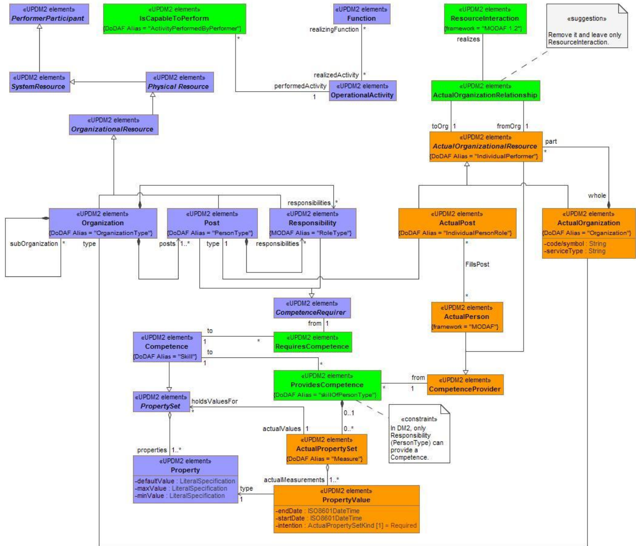
Figure A:9 - OV-4 Actual - DMM
