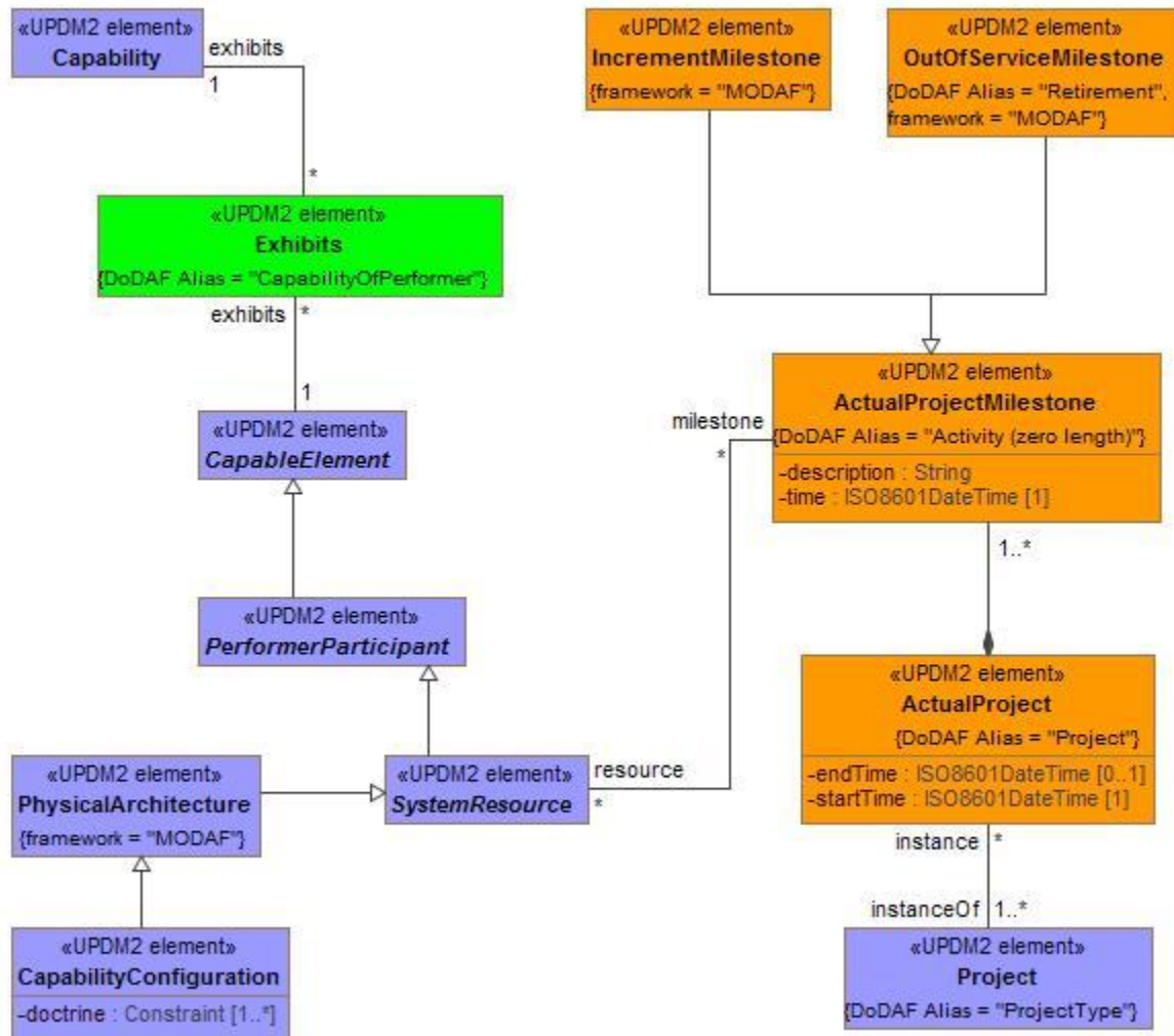
Figure A:26 - StV-3/CV-3 - DMM
