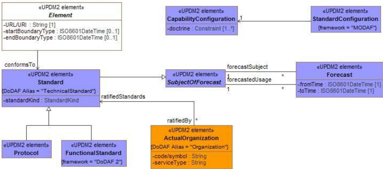
Figure A:44 - TV-1&2&3/StdV-1&2 - DMM
