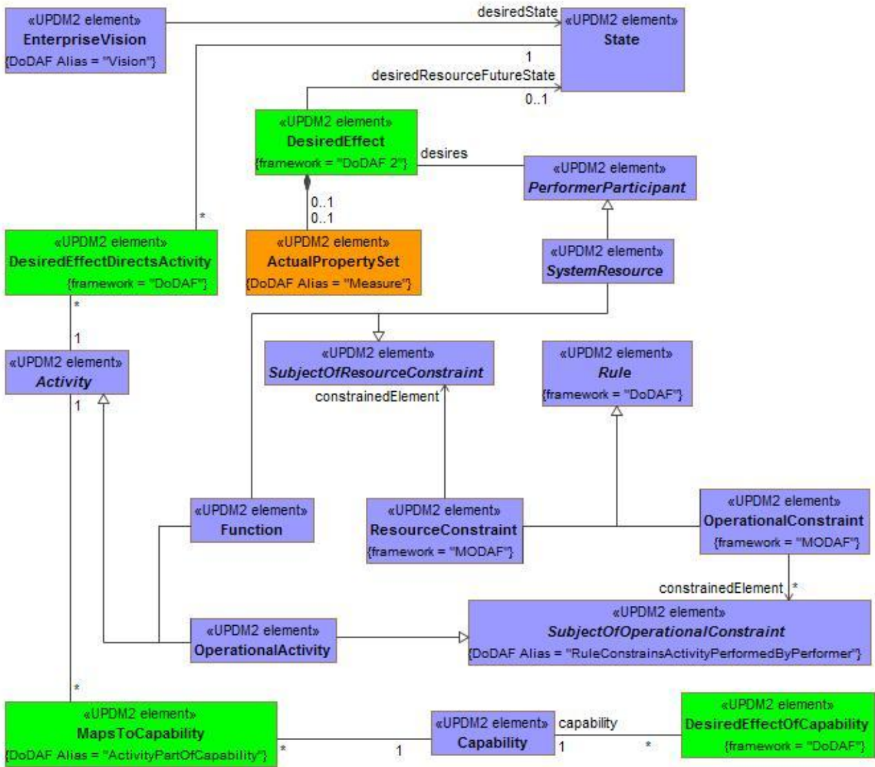
Figure A:49 - Goals - DM2
