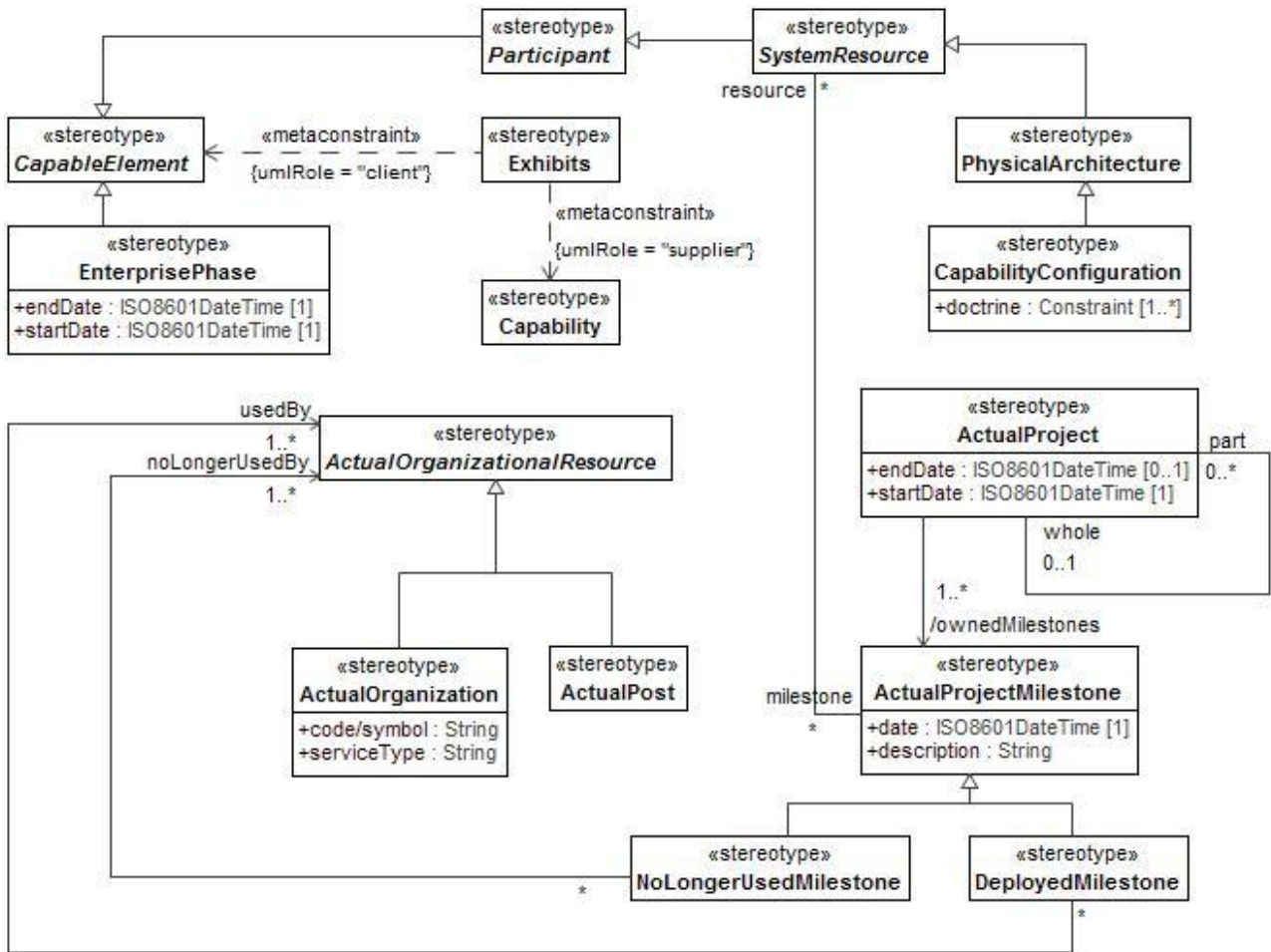
Figure B:30 - StV-5/CV-5
