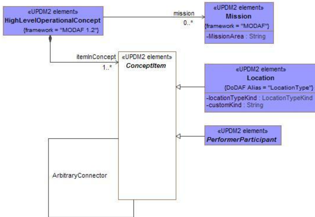
Figure A:6 - OV-1 - DMM
