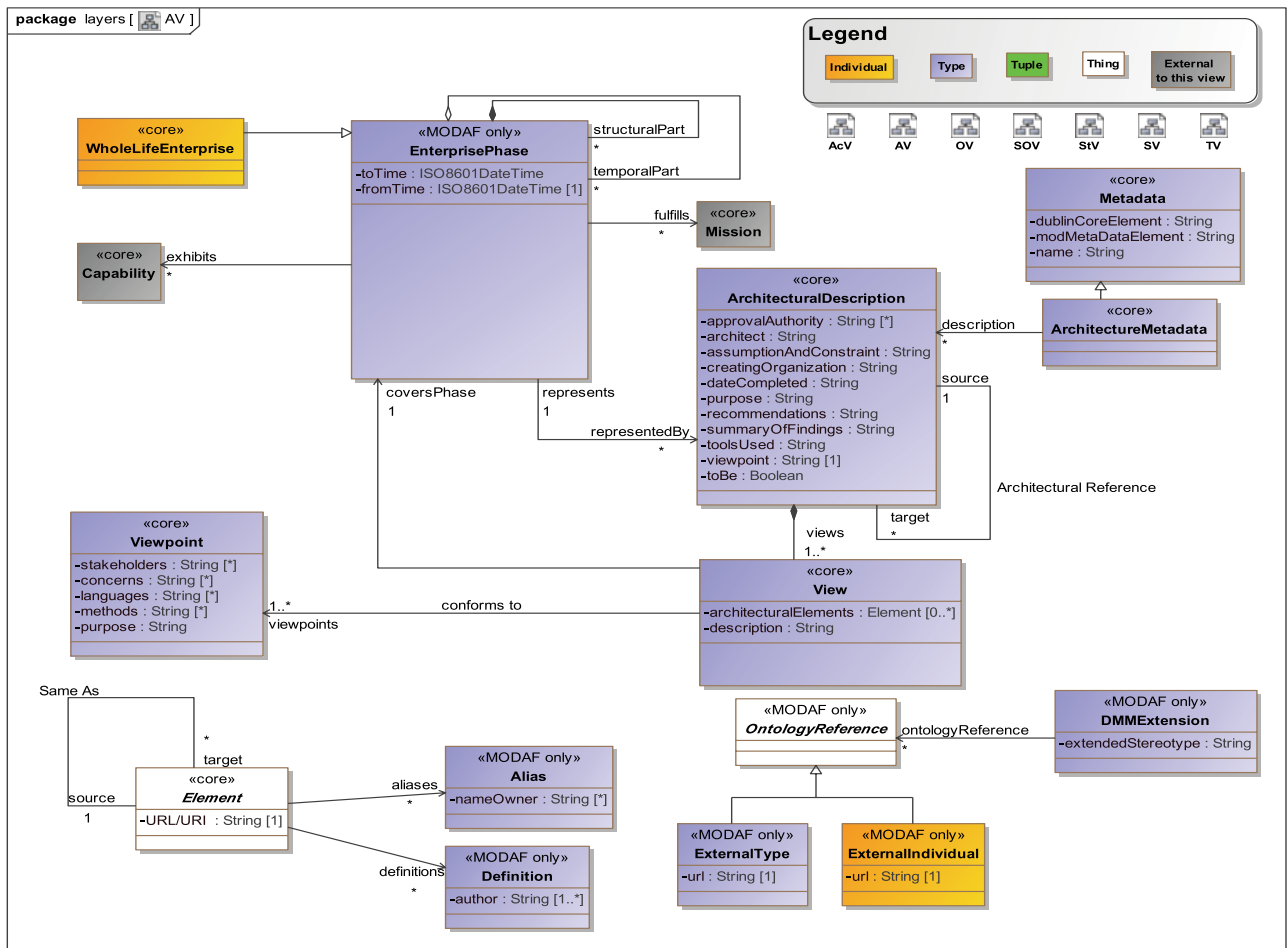
Figure A.7 - AV
