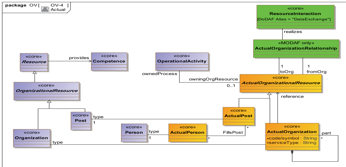
Figure A.16 - OV-4 Actual
