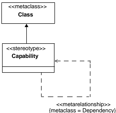
Figure 7.7 - Visualizing «metarelationship»
