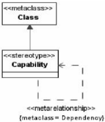
Figure 7.7 - Visualizing «metarelationship»
