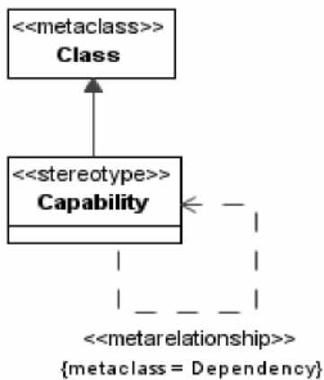
Figure 7.7 - Visualizing «metarelationship»
