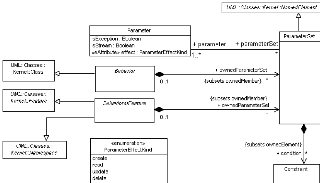
Figure 12.18 Parameter sets
