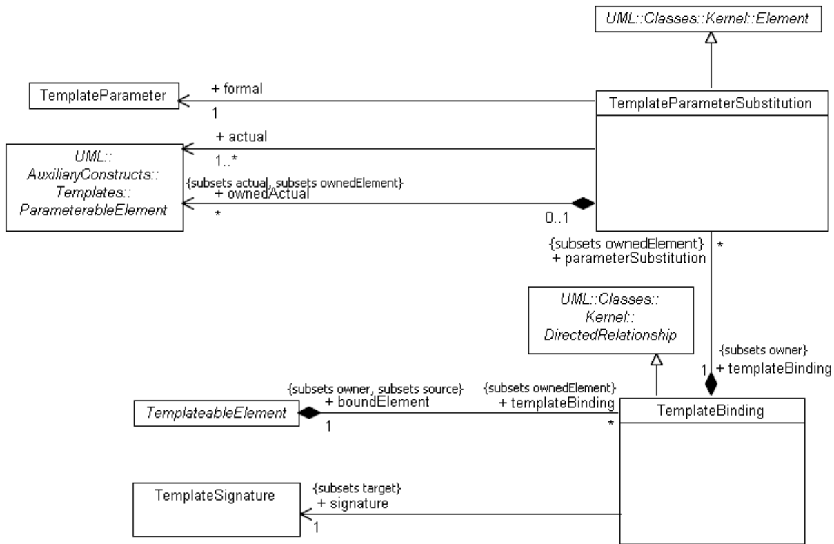
Figure 17.17 - Template parameters
