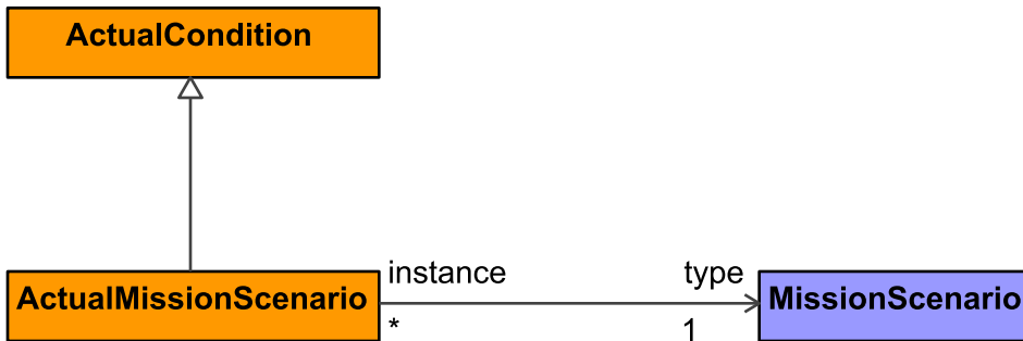
Figure 9:262 - ActualMissionScenario
