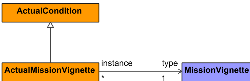
Figure 9:263 - ActualMissionVignette
