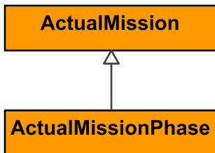
Figure 9:75 - ActualMissionPhase
