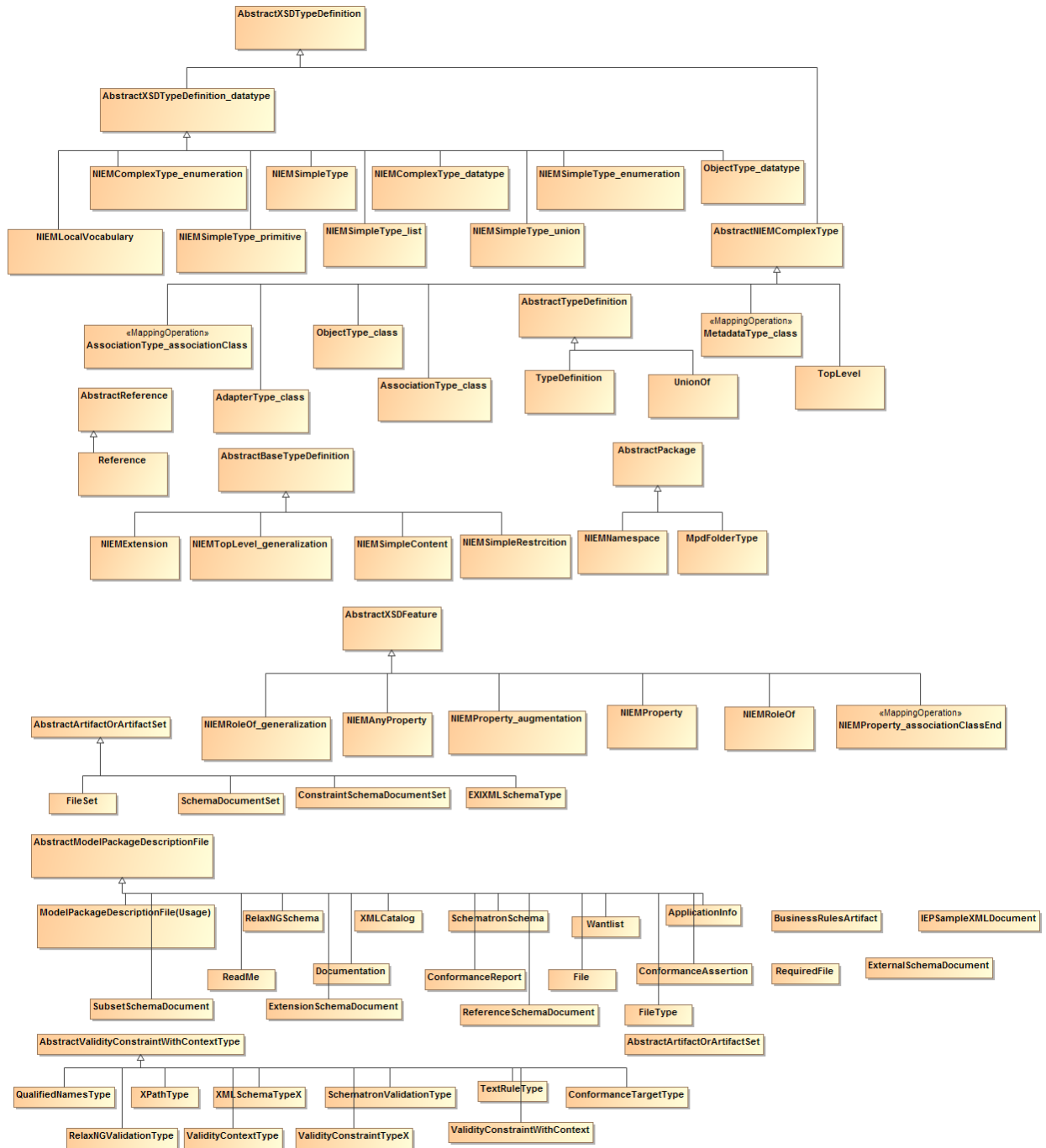
Figure 9-10 NIEM PIM to NIEM PSM Disjunction
