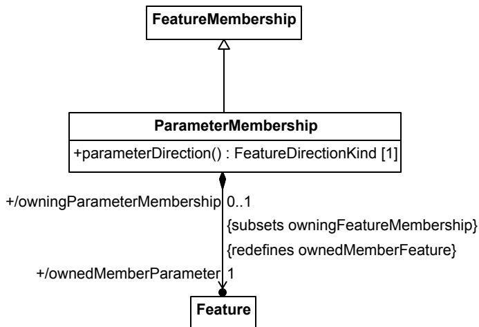
Figure 29. Parameter Memberships
