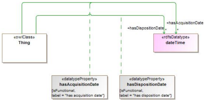
Figure 10.11 - Data Properties Numeric
