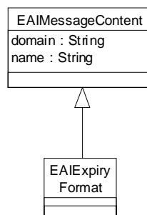
Figure 6-44 EAIExpiryFormat
