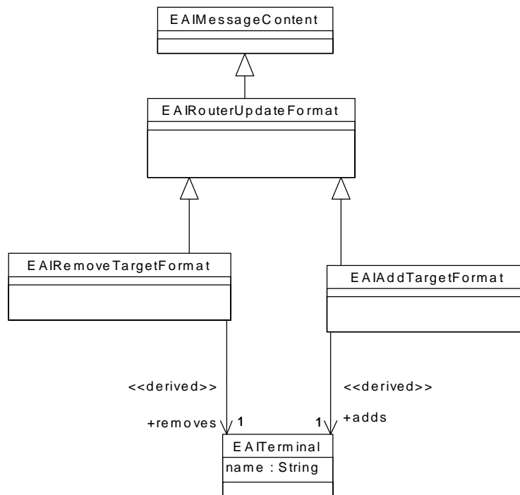
Figure 6-34 EAIRouterUpdateFormat
