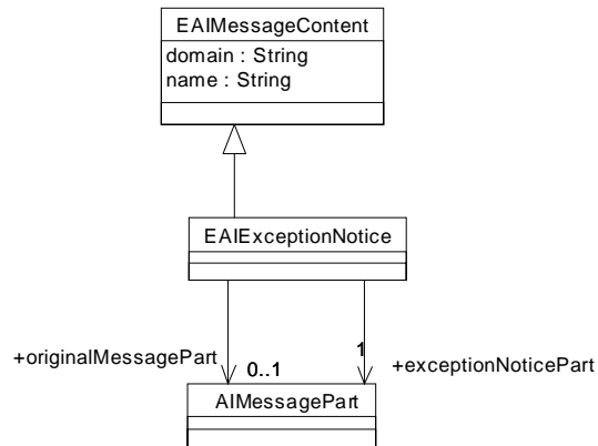
Figure 6-11 EAIExceptionNotice
