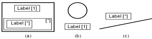
Figure A.2 - UML DI Notational Patterns
