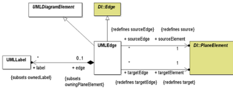
Figure A.3 - UML Edge
